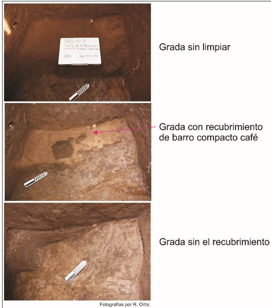
Figura 118. SAS-131. Secuencia de excavación de la grada que marca el límite Este de la Estructura 12.
