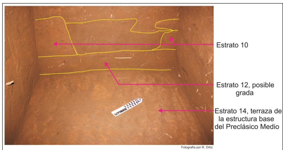
Figura 106. Detalle del Perfil Oeste de la Unidad SAS-123, que muestra la Remodelación 3 sobre el piso de la estructura base del Preclásico Medio (Estrato 10) y una posible grada (Estrato 12).
