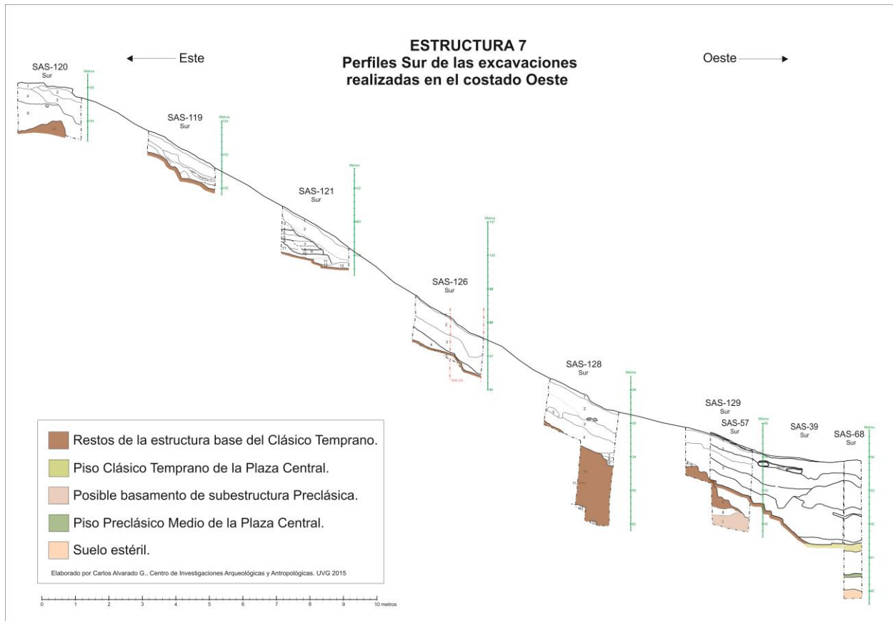
Figura 48. Perfiles Sur de 9 excavaciones realizadas en el costado Oeste de la Estructura 7.
