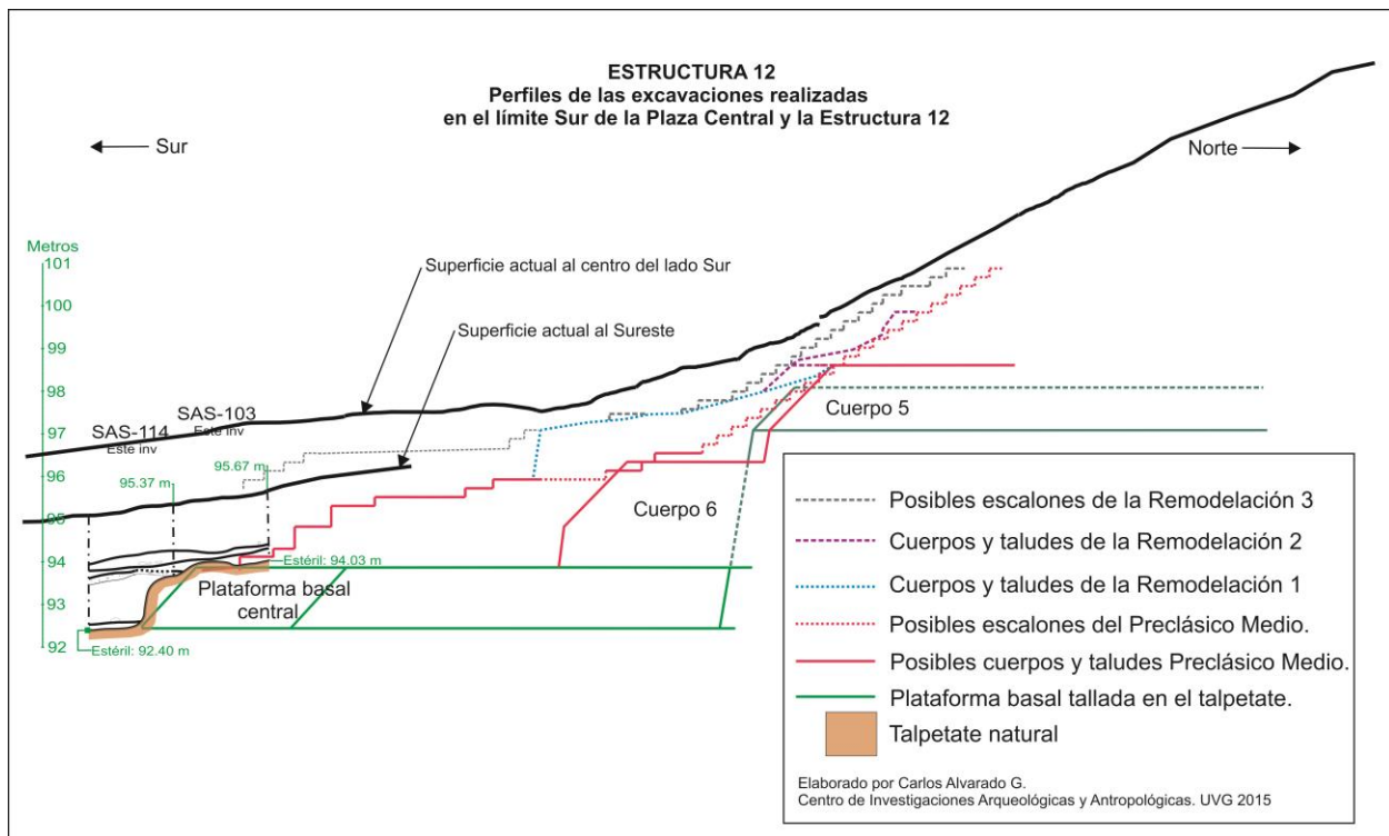
Figura 126. Corte Norte-Sur que muestra la posición de la plataforma basal tallada en el talpetate natural, identificada en SAS-103 y SAS-114.
