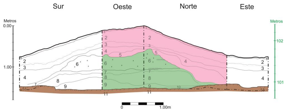
Figura 111. Perfiles de la Unidad SAS-132.
