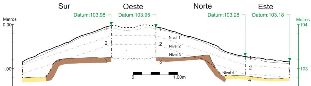
Figura 108. Terraza de la estructura base, vista al Oeste de las Unidades SAS-123 y SAS-143.
