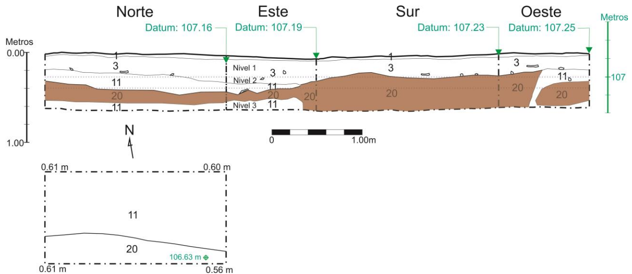
Figura 102. Unidad SAS-142. Vista de los Perfiles Oeste, Norte y Este.
