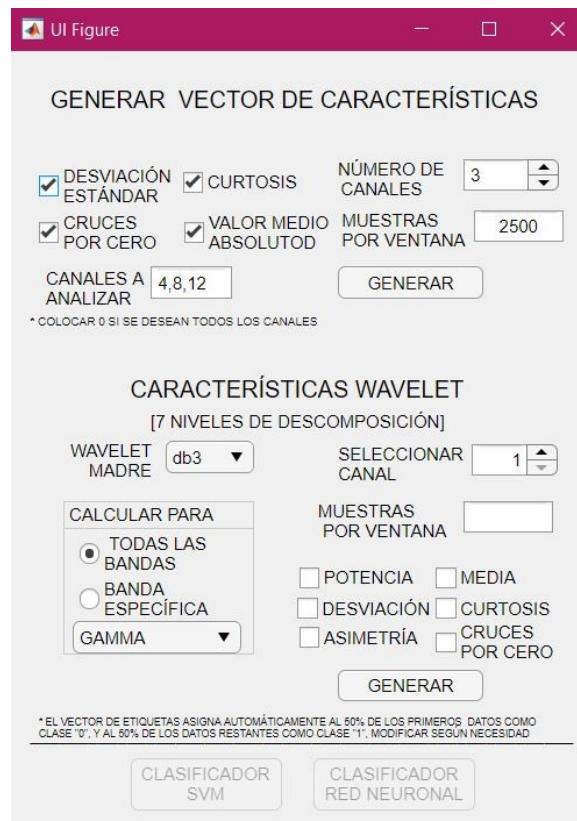
Figura 23: Ventana de extracción de características de la señal EEG.
