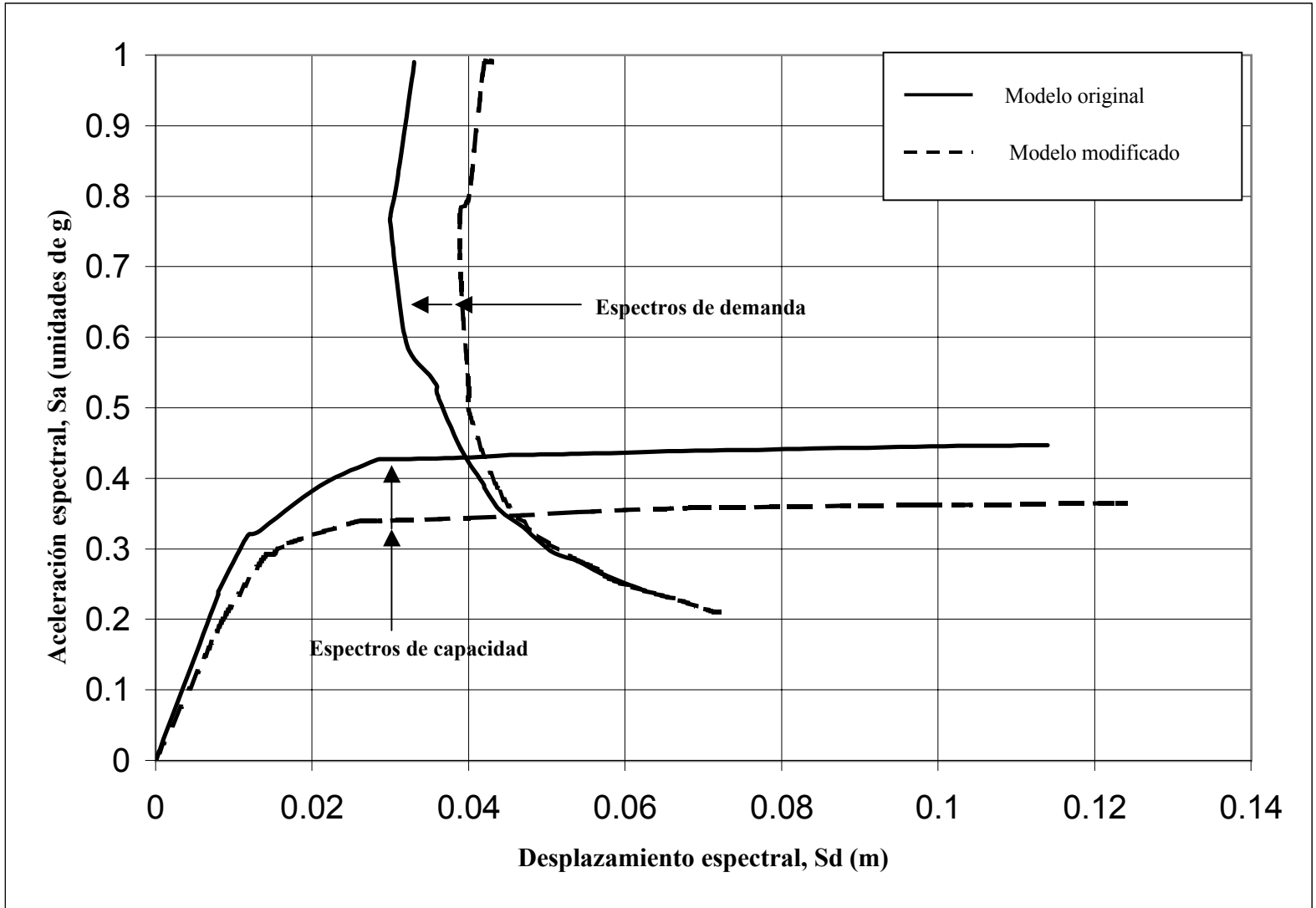
Figura 60: Espectros de capacidad y demanda del modelo original y modelo modificado, carga dirección "y"
