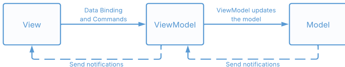
Figura 5.2. Diagrama de relaciones de los componentes MVVM
