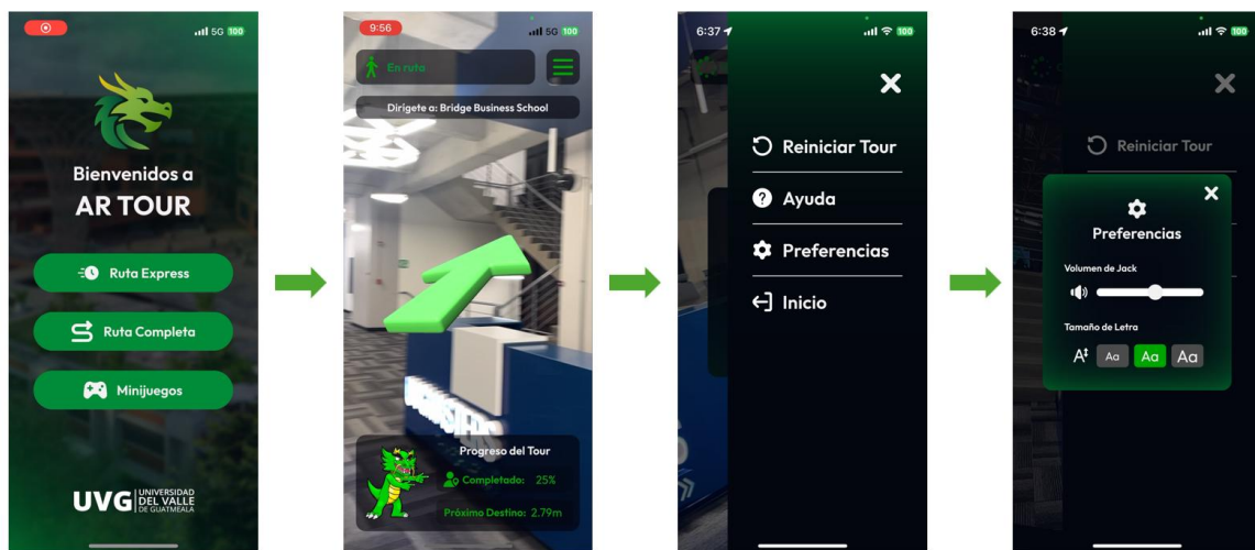
Figura 7.4. Secuencia de pantallas del sistema de interfaz de usuario
