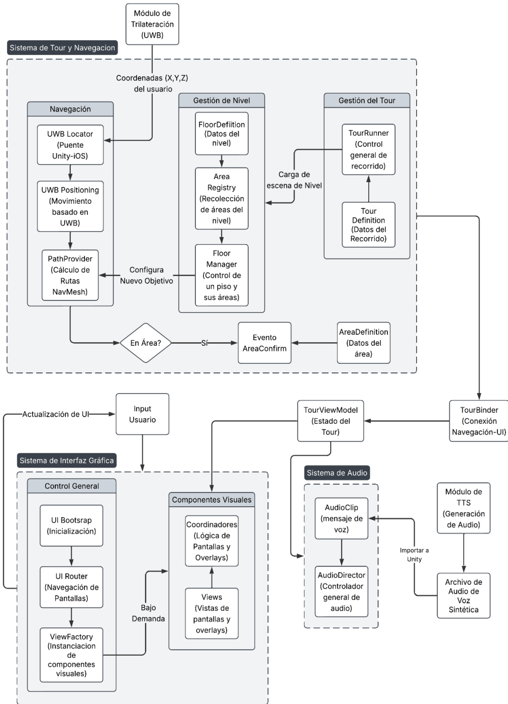
Figura 6.1. Diagrama de arquitectura general de la aplicación
