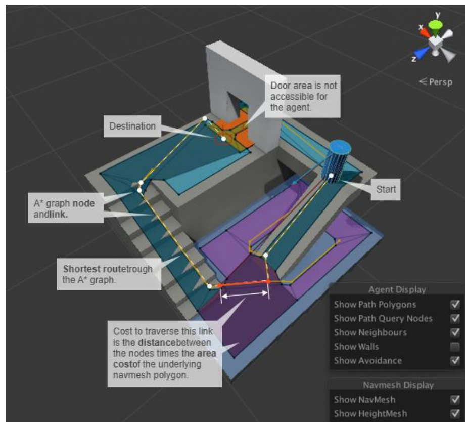
Figura 5.3. Ejemplo de áreas y costos de NavMesh en Unity
