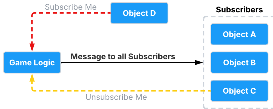
Figura 5.1. Diagrama del Patrón Observador
