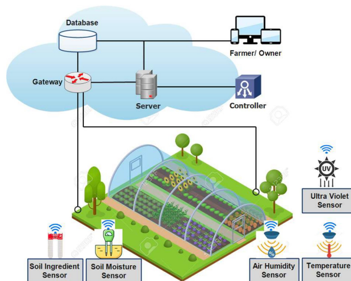
Figura 1: Esquema de un sistema IoT aplicado a la Agricultura 4.0, donde los sensores de campo recopilan datos ambientales y del suelo, los cuales se envían a una plataforma en la nube para su análisis y control remoto.
