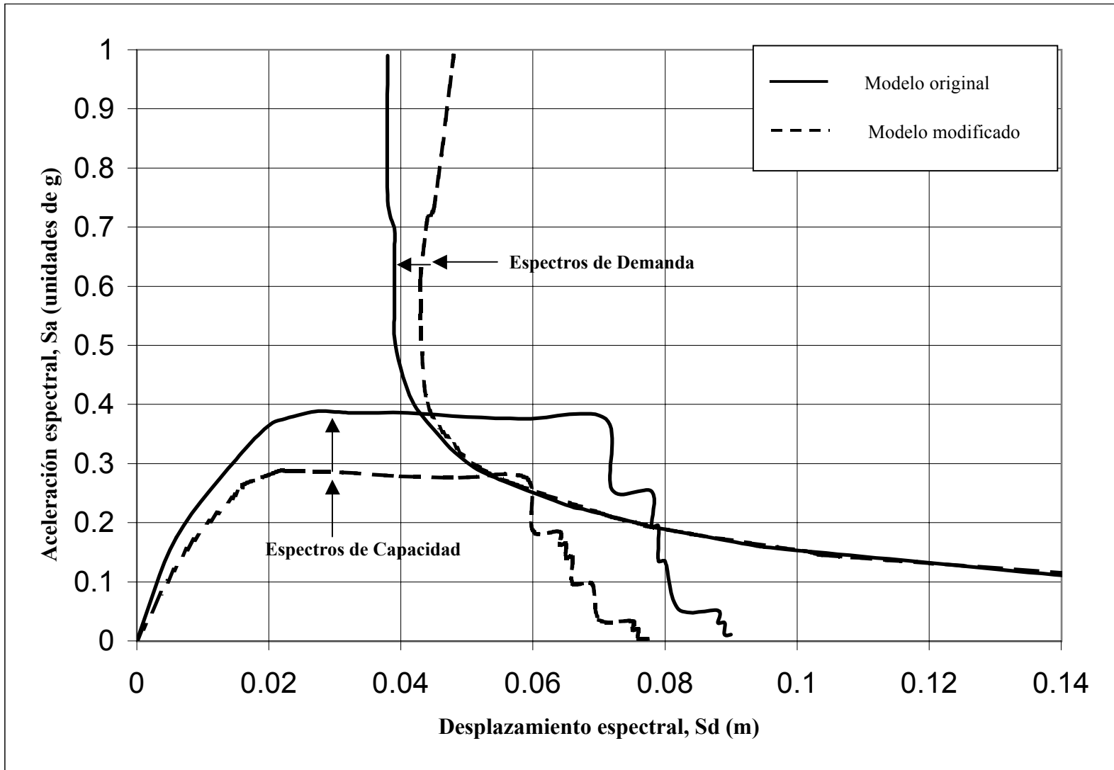
Figura 59: Espectros de capacidad y demanda del modelo original y modelo modificado, carga dirección "x"
