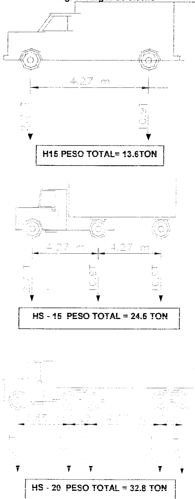
Fig. 3: Cargas de diseño
