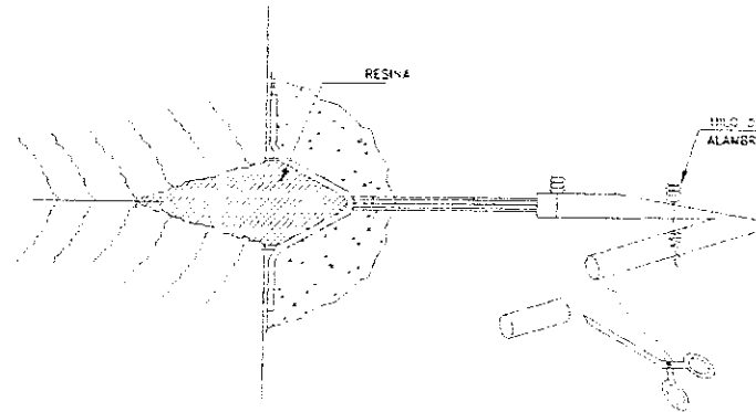
Fig. 12.4 : Continuación inyección de grietas
