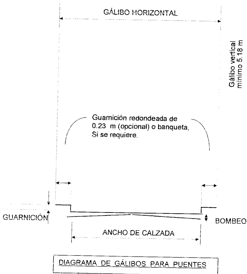
Fig. 2 : Diagrama de gálibos para puentes
