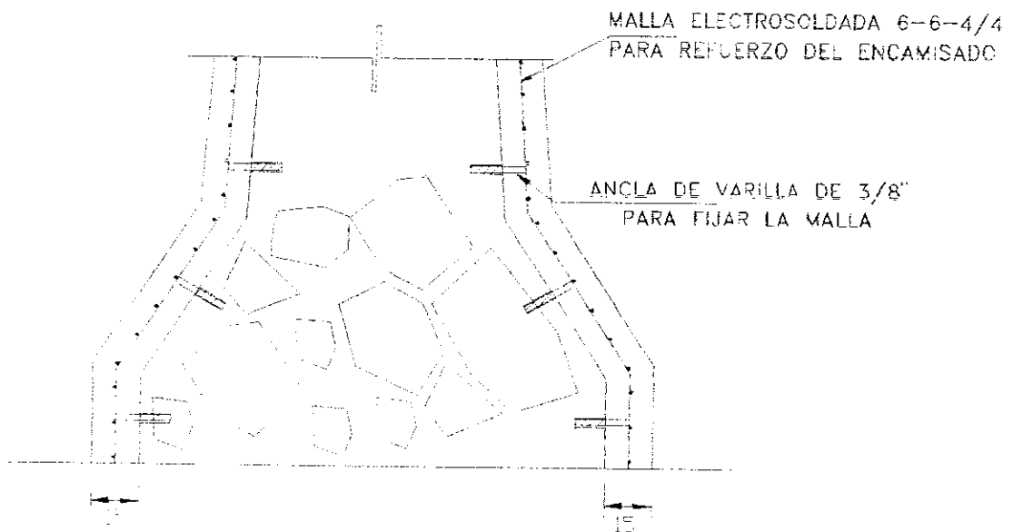
Fig. 14.4 : Continuación encamisado de pilas
