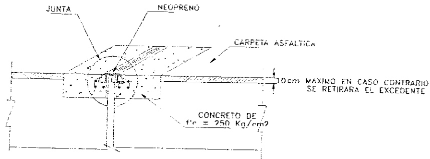
Fig. 13.1 : Continuación cambio de juntas de dilatación
