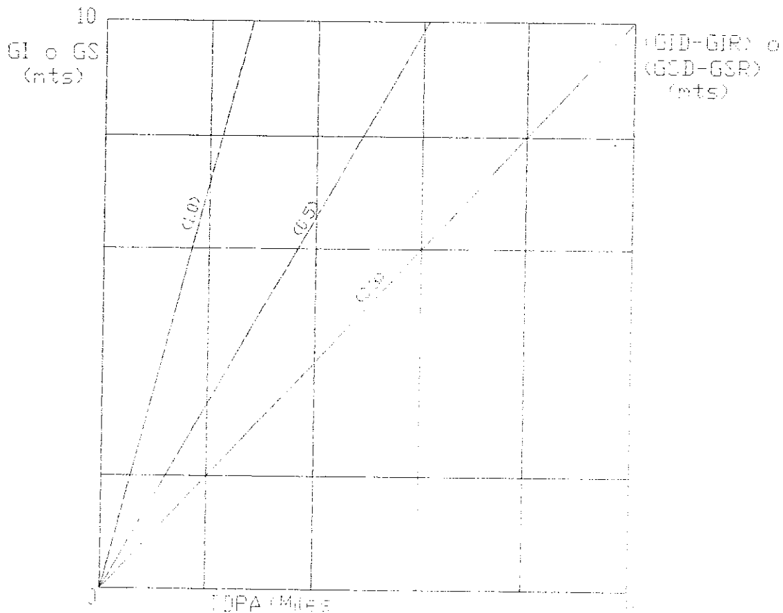
Fig. 9: Gráfica de GI contra TPDA para diferentes valores de GID-GIR
