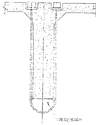
Fig. 16 : Continuación tipos del preesfuerzo exterior
