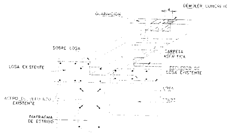
Fig. 13 : Cambio de juntas de dilatación
