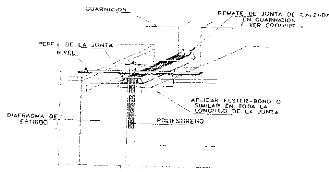
Fig. 13.3 : Continuación cambio de juntas de dilatación
