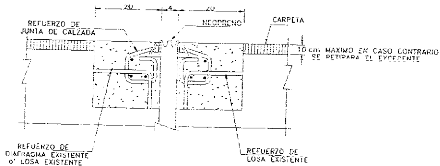
Fig. 13.2 : Continuación cambio de juntas de dilatación
