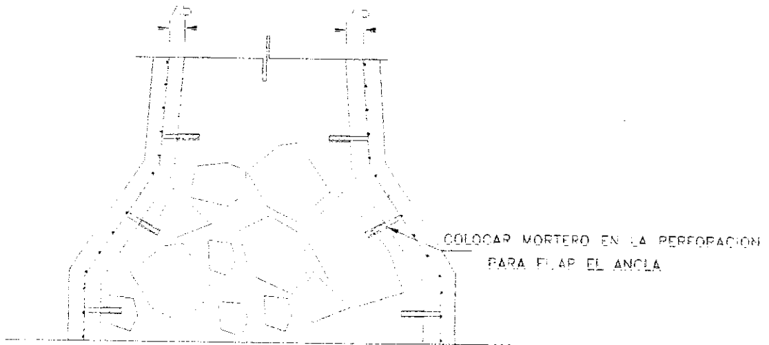
Fig. 14.3 : Continuación encamisado de pilas
