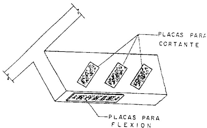
Fig. 15 : Refuerzo con placas y perfiles metálicos
