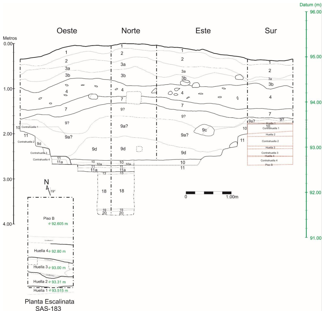
UNIDAD SAS-183 Proyecto Arqueológico Semetabaj 2017 Original: Pablo Estrada Digitalización: Carlos Alvarado G.
