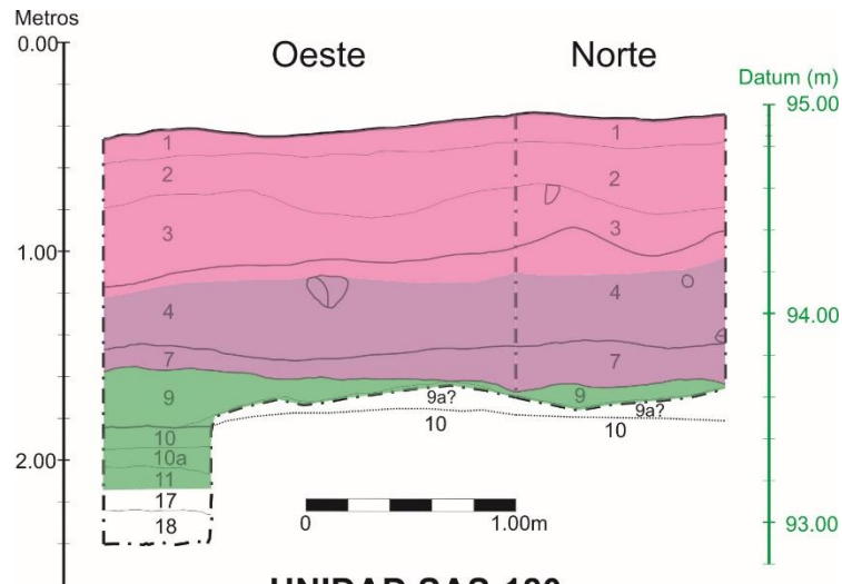
UNIDAD SAS-180 Proyecto Arqueológico Semetabaj 2017
