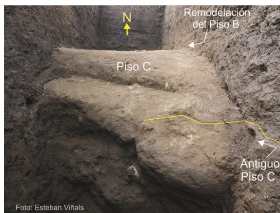
Figura 26. Unidad SAS-197. Vista en perfil del límite Sur de la terraza del Piso C.
