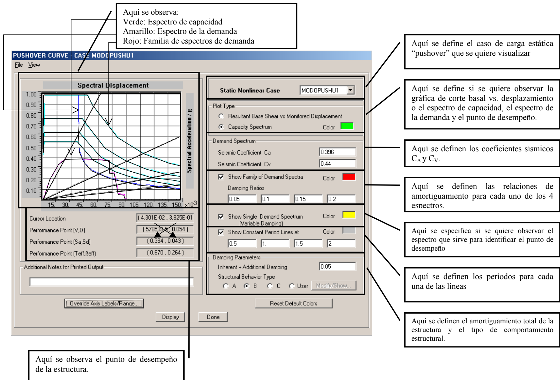
Figura 47: Ventana de espectro de capacidad, espectro de demanda y punto de desempeño
