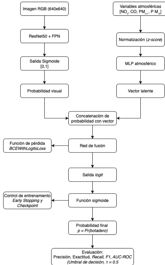
Figura 1: Flujo general del algoritmo multimodal para estimar la probabilidad de presencia de botadero a cielo abierto
