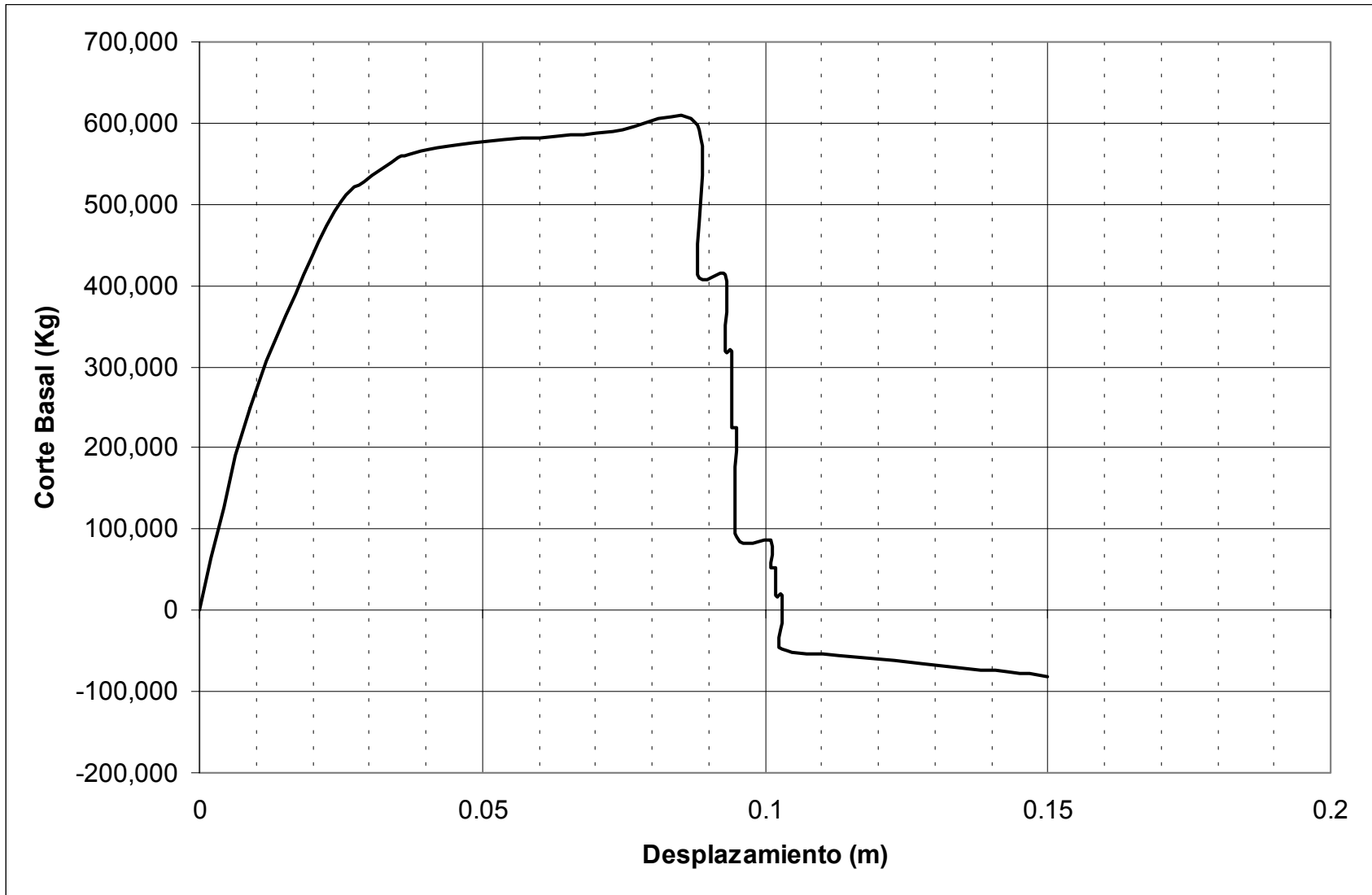
Figura 43: Gráfica de corte basal vs. desplazamiento del caso de carga estática "pushover" en la dirección "x"
