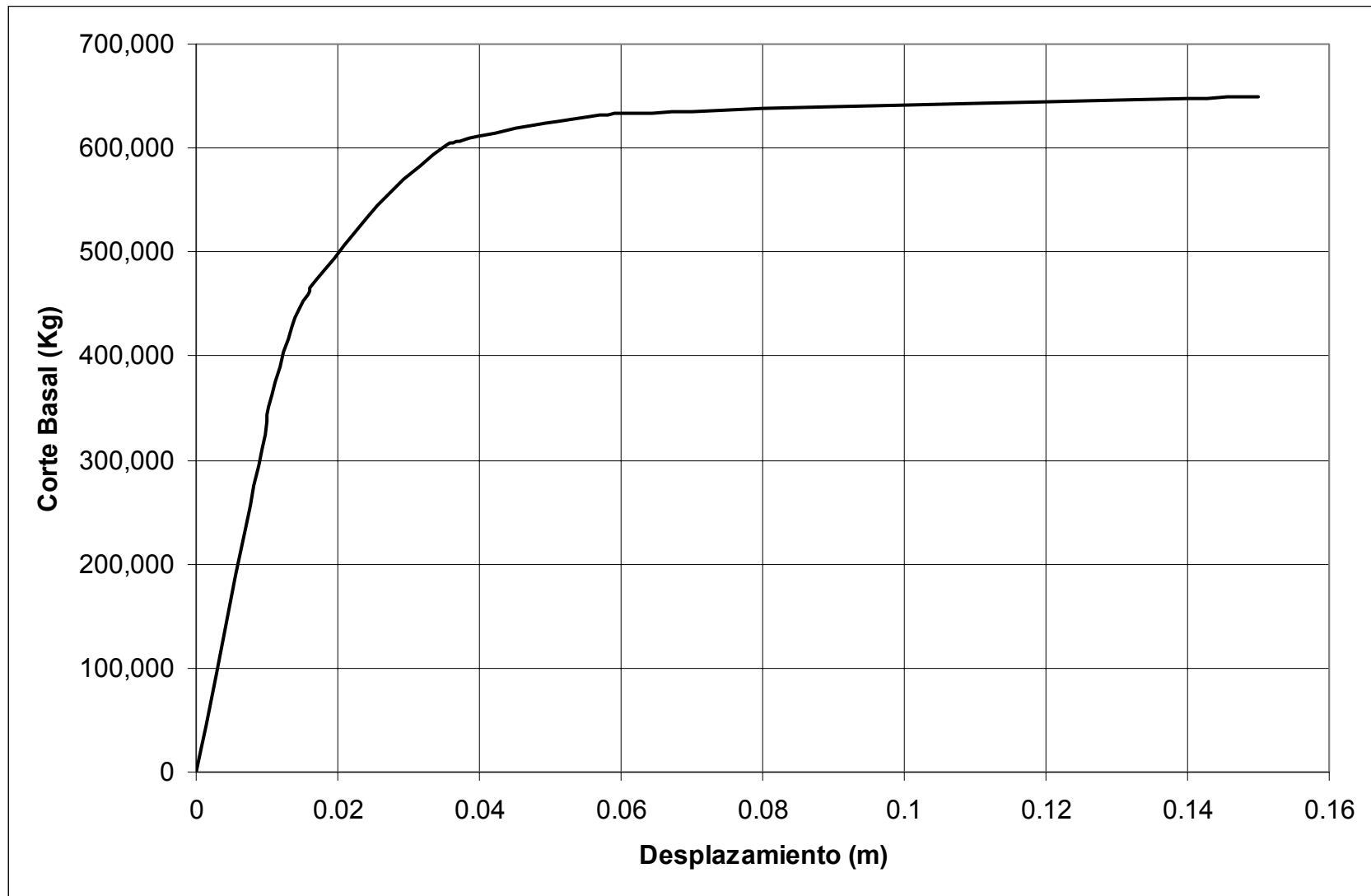
Figura 44: Gráfica de corte basal vs. desplazamiento del caso de carga estática "pushover" en la dirección "y"
