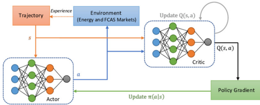
Figura 5: Arquitectura PPO con DRL [22]
