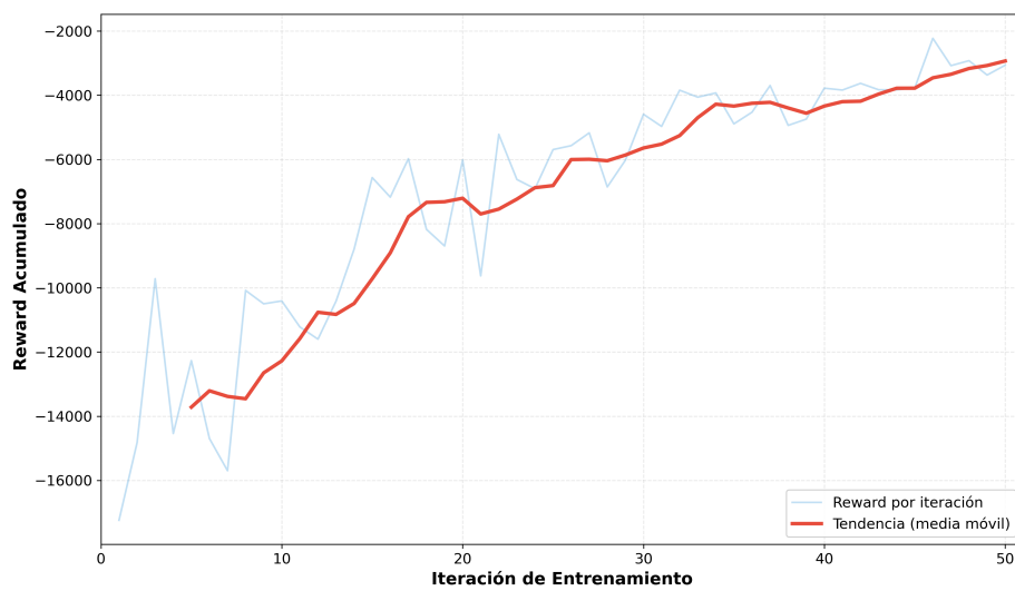
Figura 17: Curva de aprendizaje en Avenida Reforma
